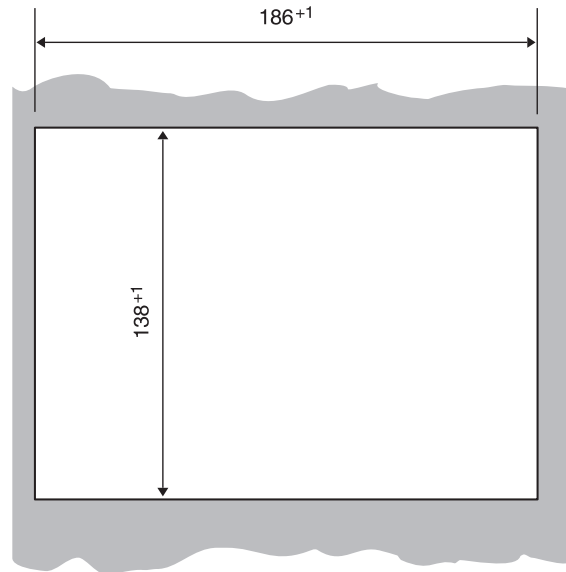
Ausschnitt Schaltschranktür
