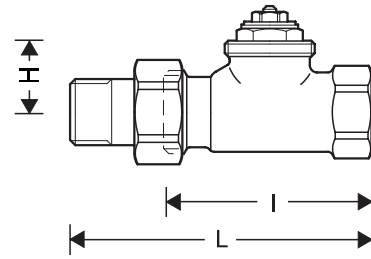
Abb. 6. Durchgang
