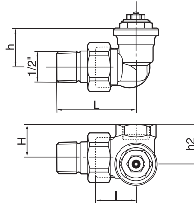
Abb. 8. Winkeleck
