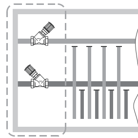
Kombi-3-Plus - Verteiler
